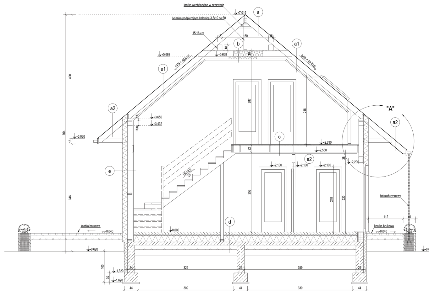
PRZEKRÓJ A-A 1:50
